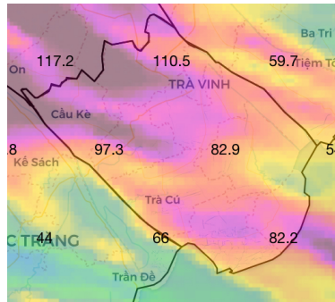
Bảng đồ dự báo mưa 24h tới
